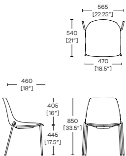
OLA/1 Four Leg Non Arm
