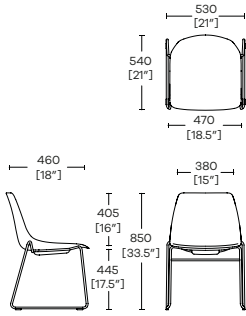
OLA/2 Sled Non Arm
